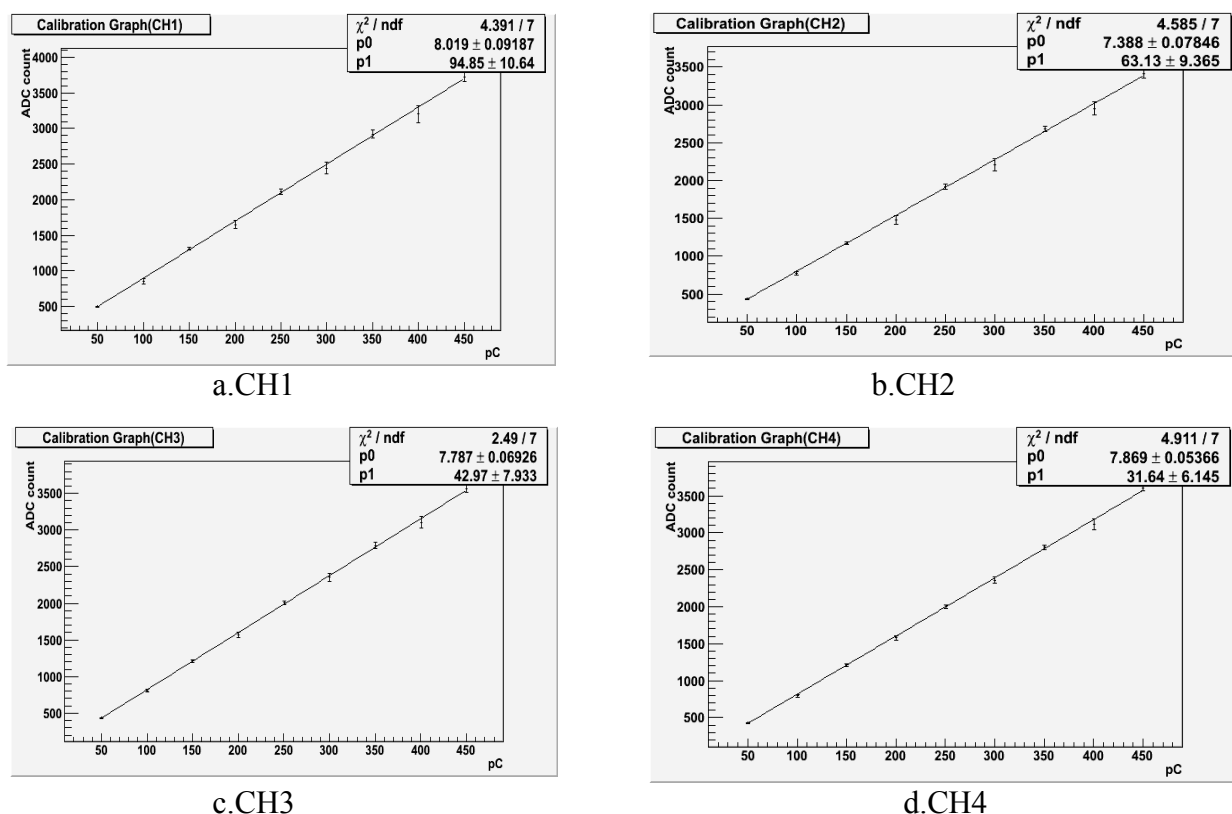
図 3.3.2 各チャンネルの測定結果
