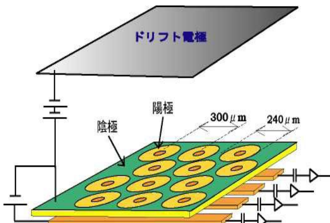
図 1.2.1 \mu -PIC の構造[4]
