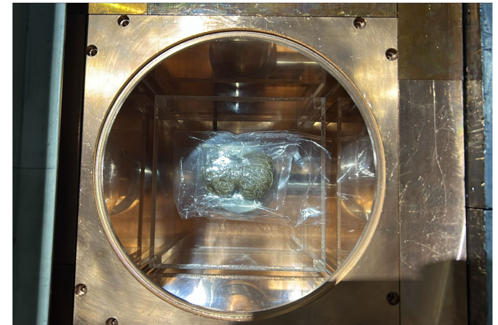
ゲルマニウム検出器
